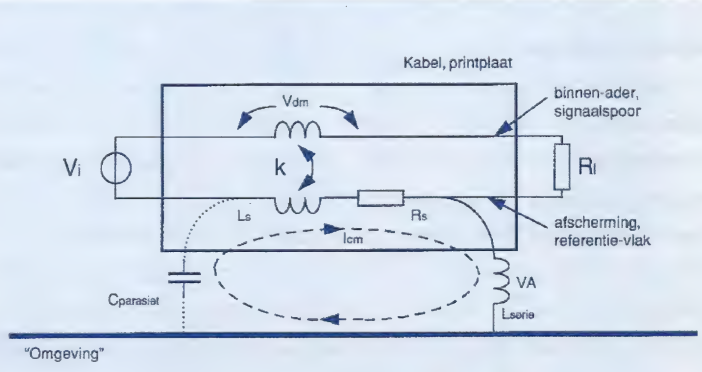
Figuur 7 Transfer impedantie, CM stroom naar DM spanning omzetting
